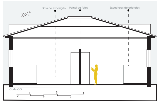
Corte museu
