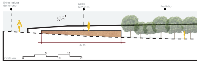
Corte da topografia
