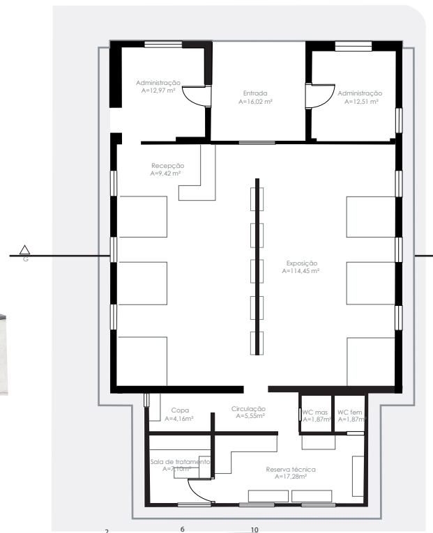
Planta museu
