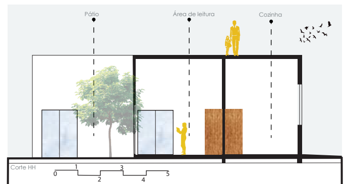
Corte Casa Mirante
