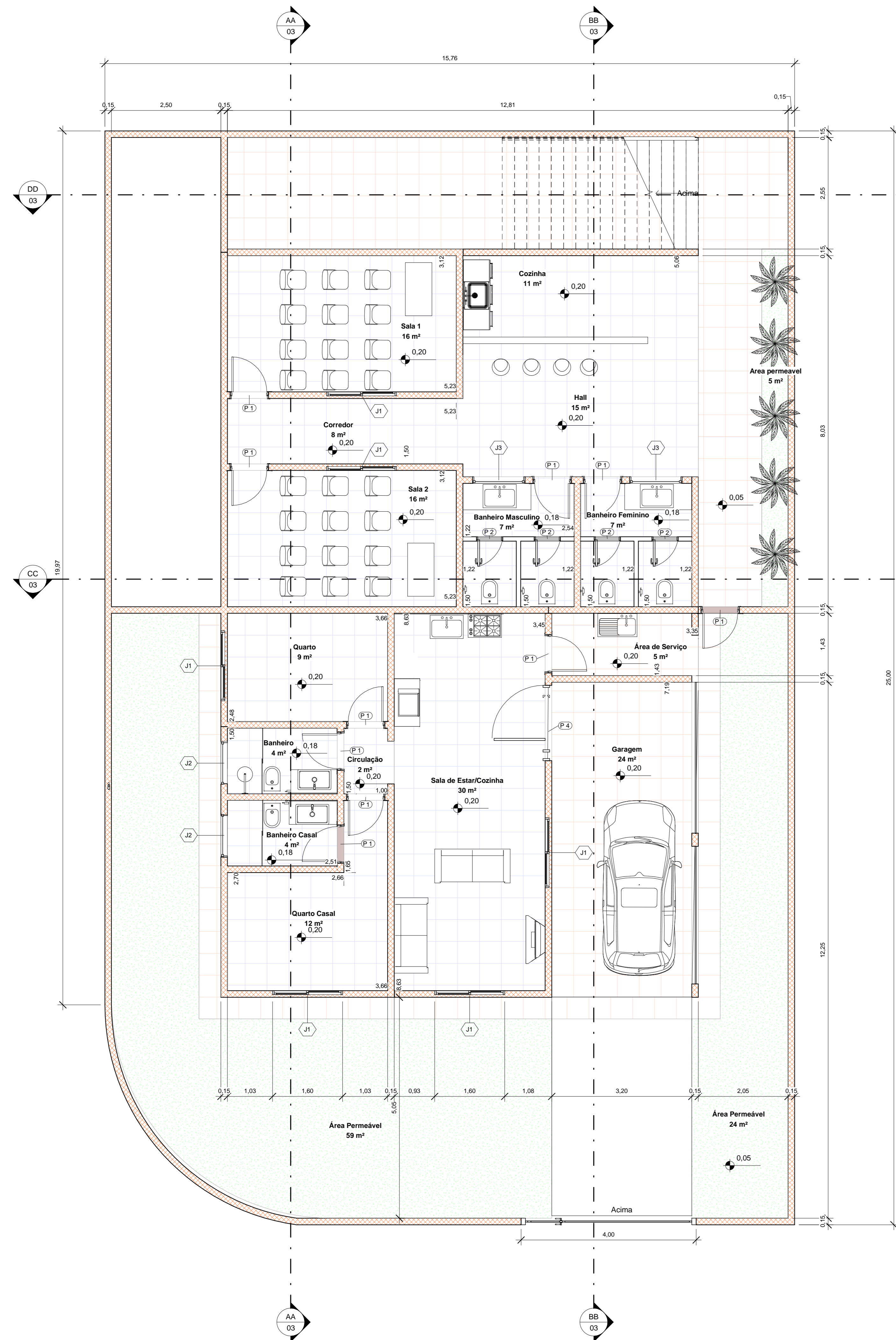
1 Pav. Térreo 1 : 50
