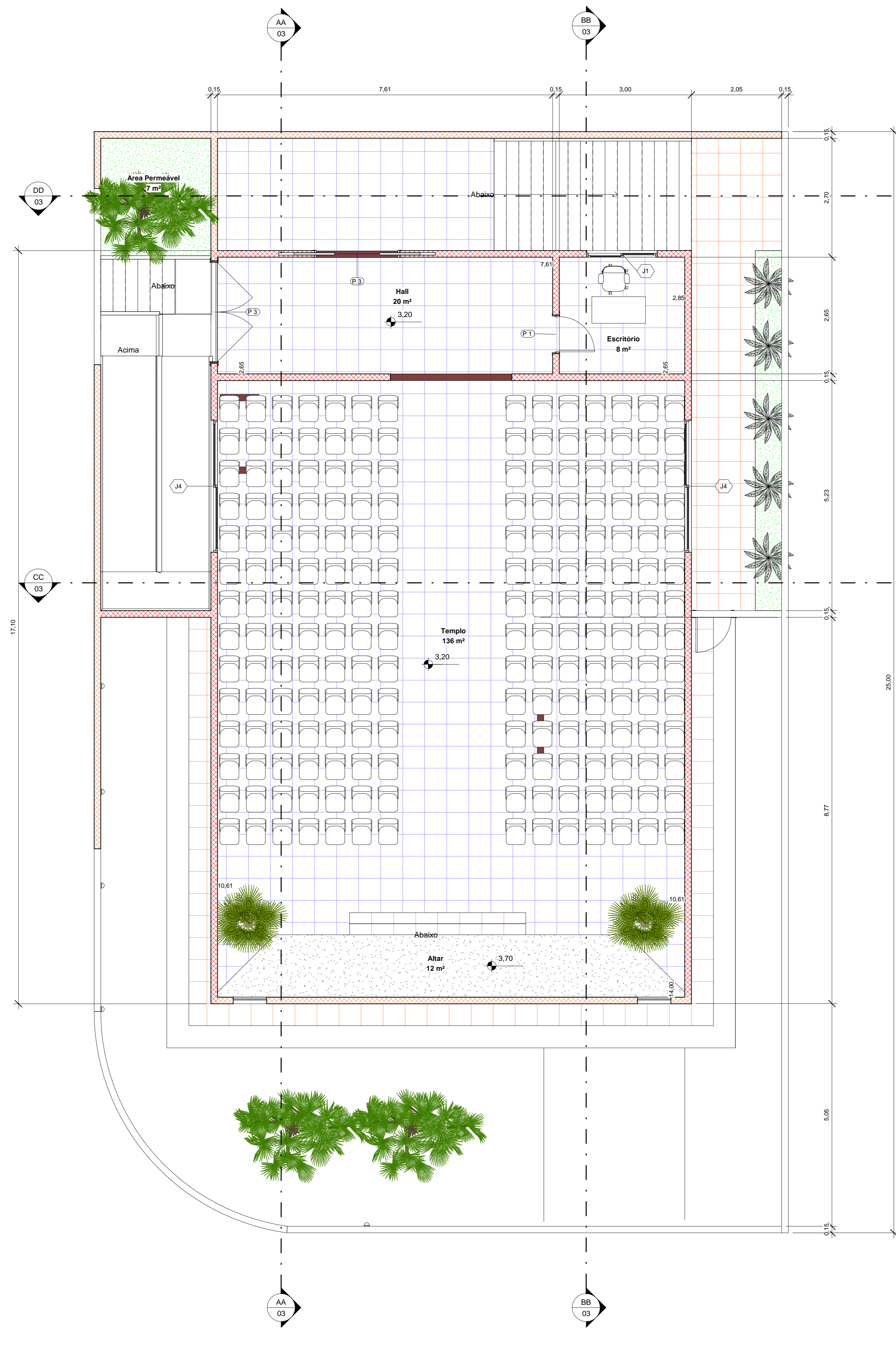
2 Pav. Superior 1 : 50
