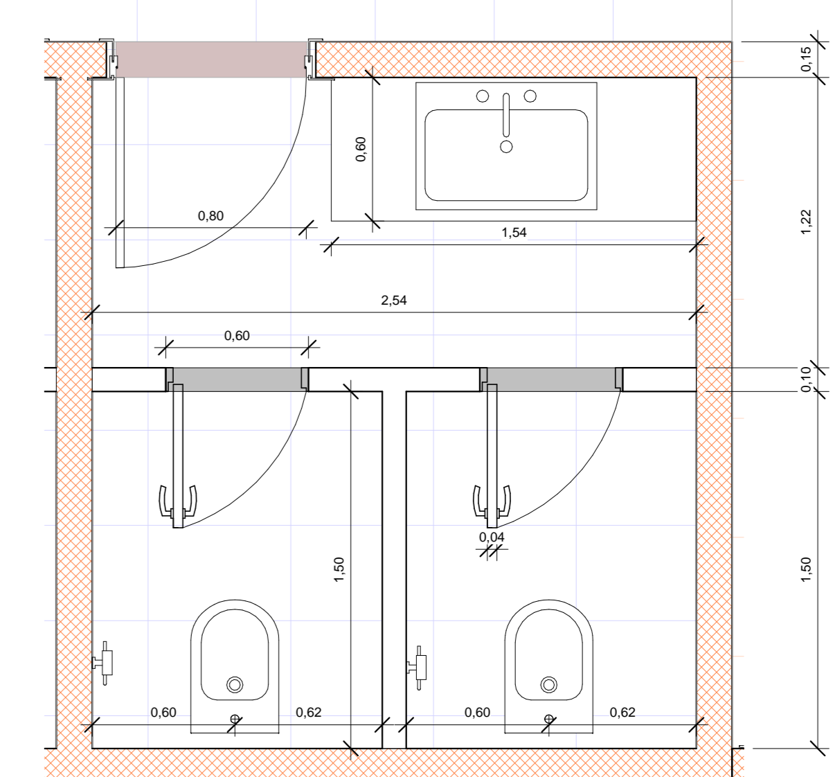
3 Detalhe - Banheiro 1 : 20
