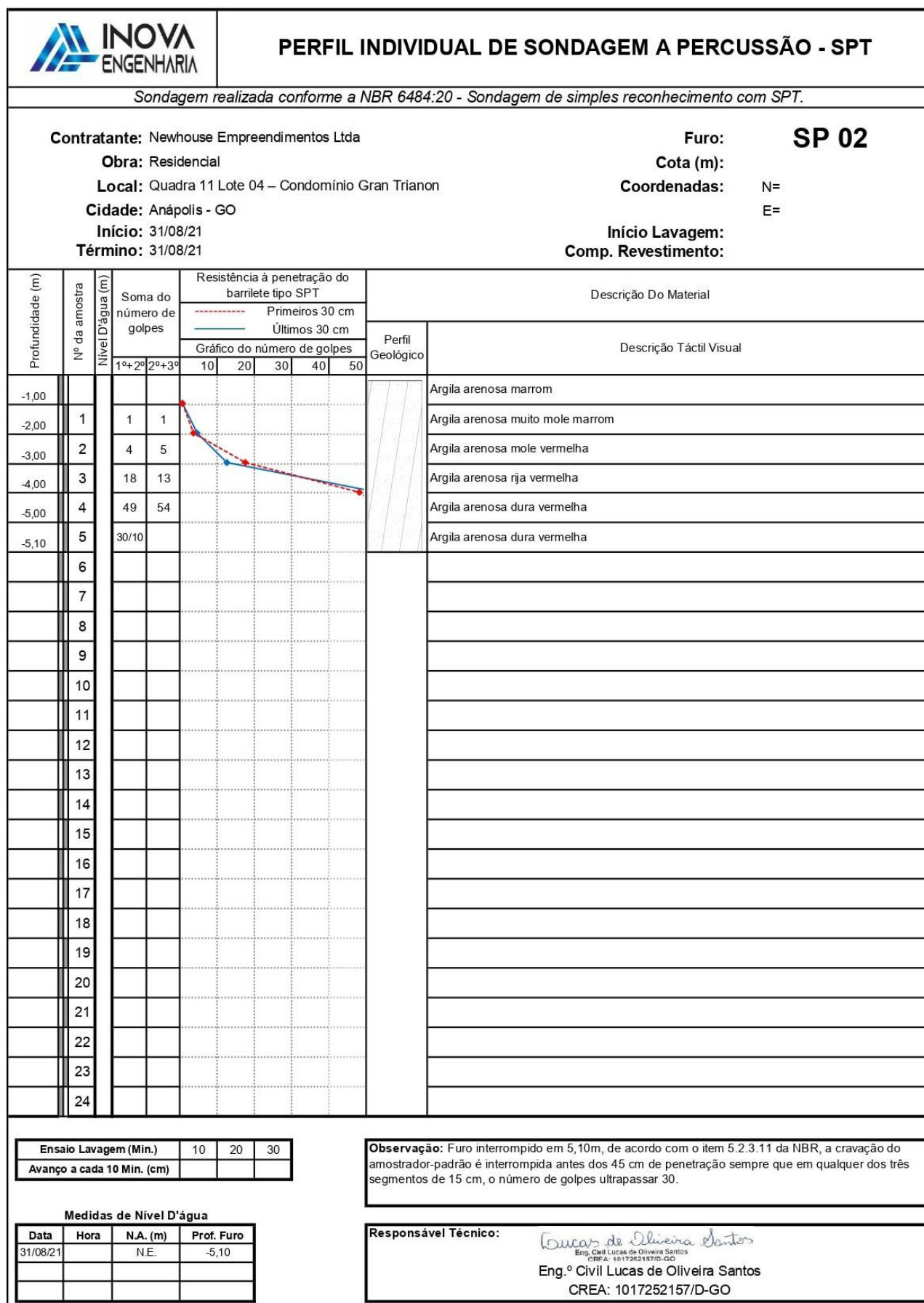
Figura 20 - Perfil individual de sondagem do ensaio SPT
