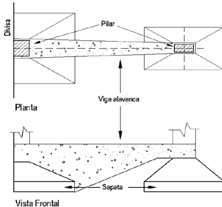
Figura 6 - Sapata de divisa.
