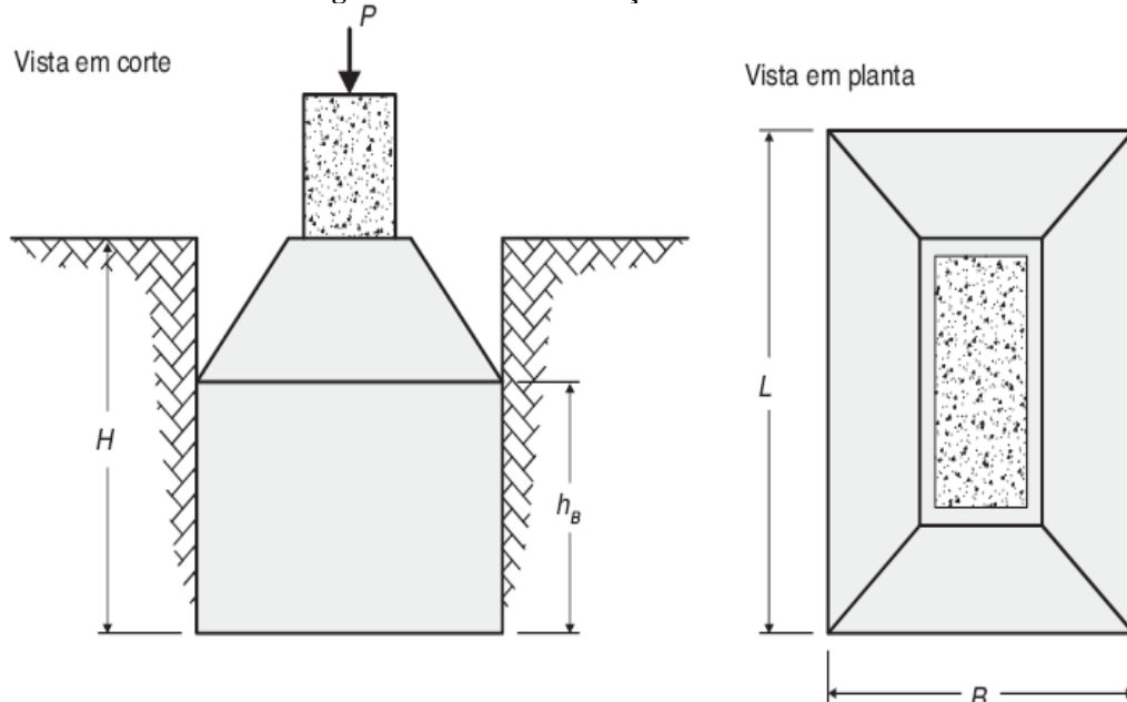
Figura 7 - Bloco de fundação convencional
