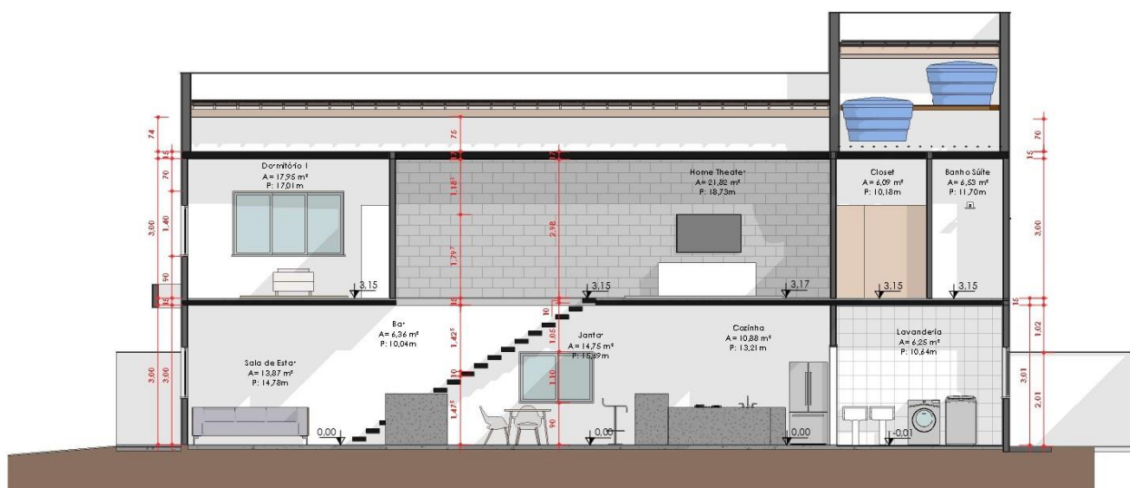
Figura 18 - Corte BB
