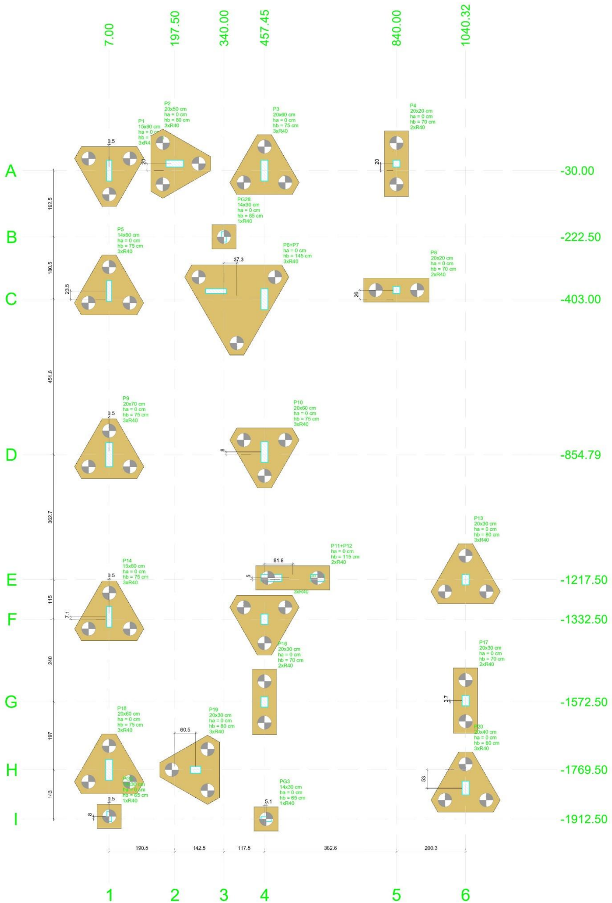
Figura 24 - Planta de locação estacas
