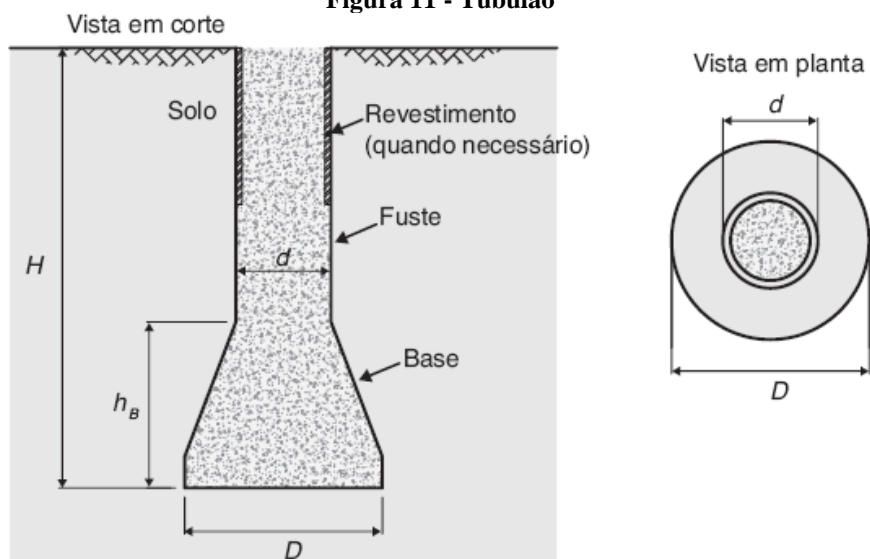
Figura 11 - Tubulão
