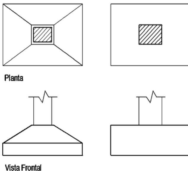
Figura 3 - Sapata isolada
