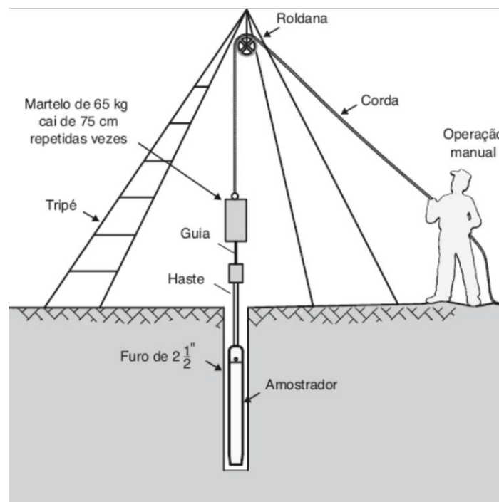
Figura 1 - Ensaio a percussão SPT
