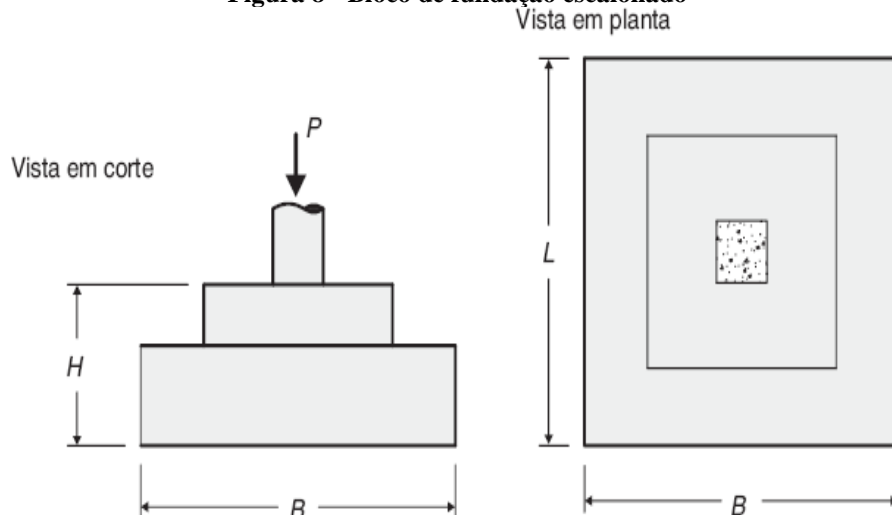
Figura 8 - Bloco de fundação escalonado
