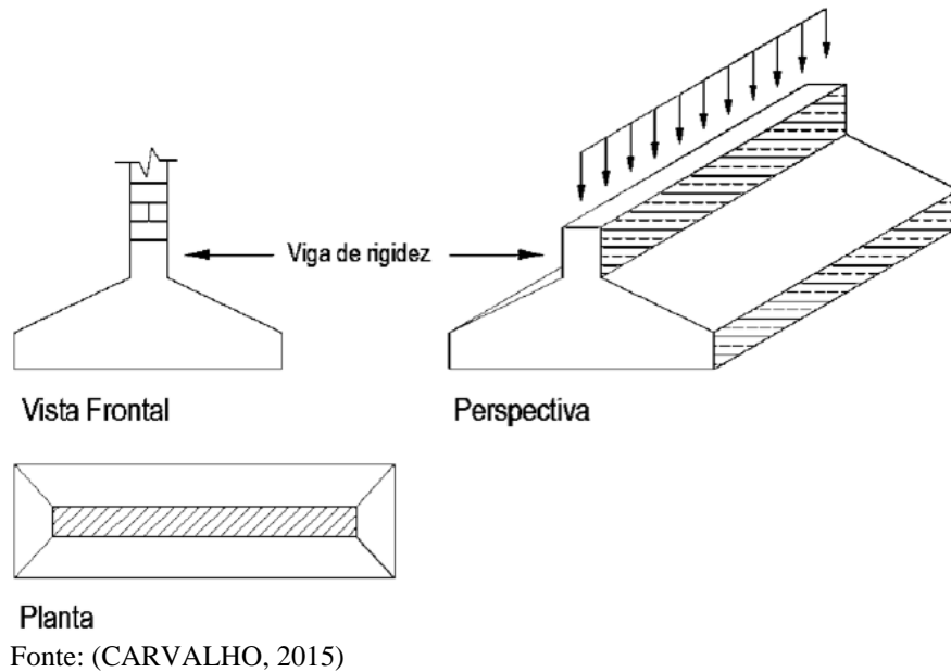
Figura 4 - Sapata corrida sob carregamento linear distribuído
