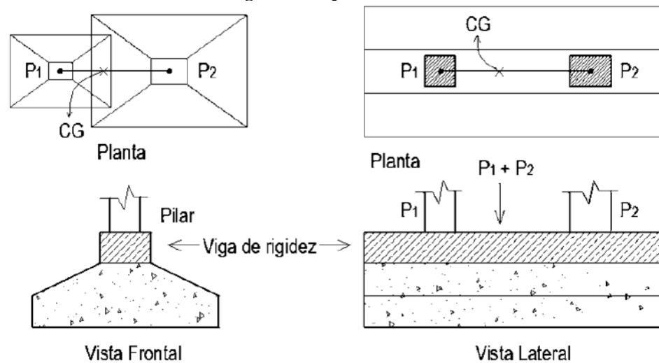
Figura 5 - Sapata associada
