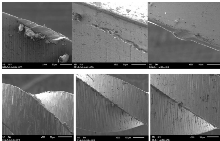
Figura 3. Exemplificação das falhas encontradas na superfície ativa dos instrumentos em ambos os grupos experimentais analisados; Sistema Biorace® e Sistema Protaper Next®
