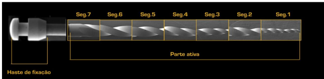
Figura 2. Ilustração em imagem de MEV do lado A do instrumento Protaper Next® caracterizando as áreas de análises de falhas (50x).
