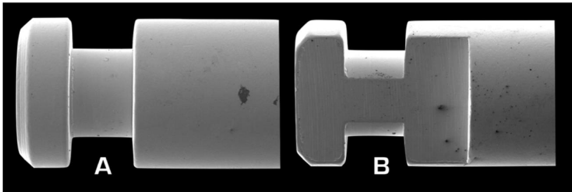
Figura 1. Imagem em 50x (MEV) da haste de fixação do instrumento de NiTi (lados A e B).
