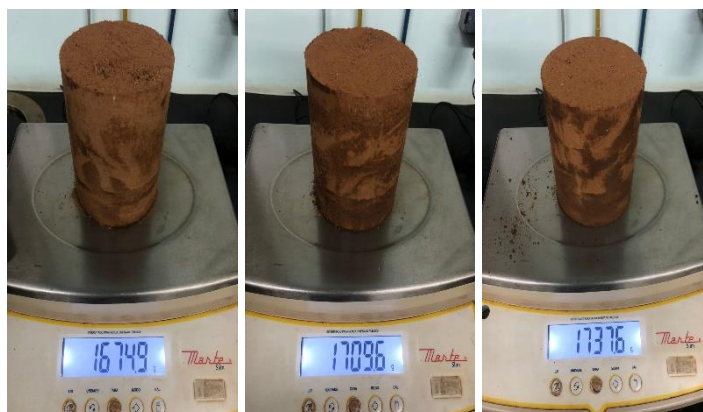
Figura 9 - Ensaio de Compactação (Corpos de Prova)
