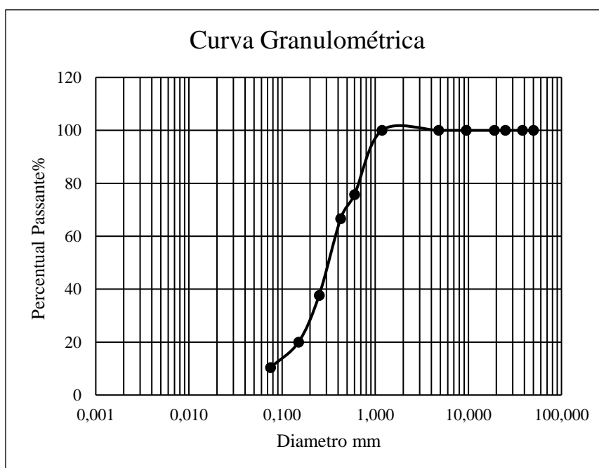
Figura 4 - Curva Granulométrica
