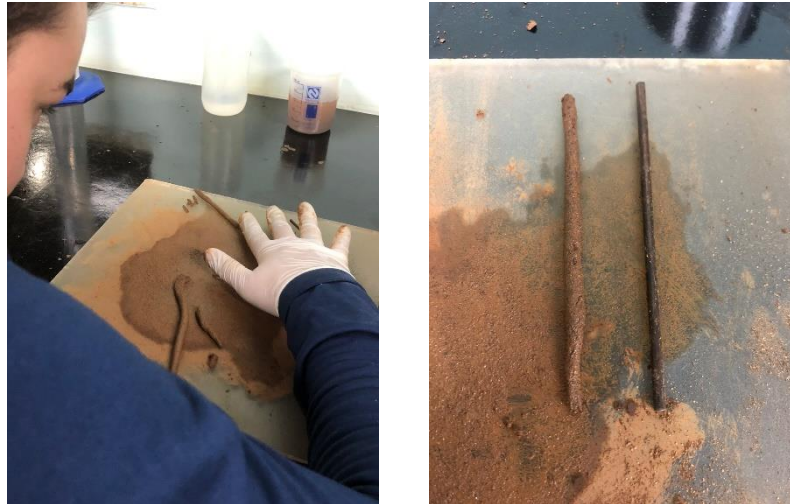
Figura 6 - Ensaio de Limite de Plasticidade
